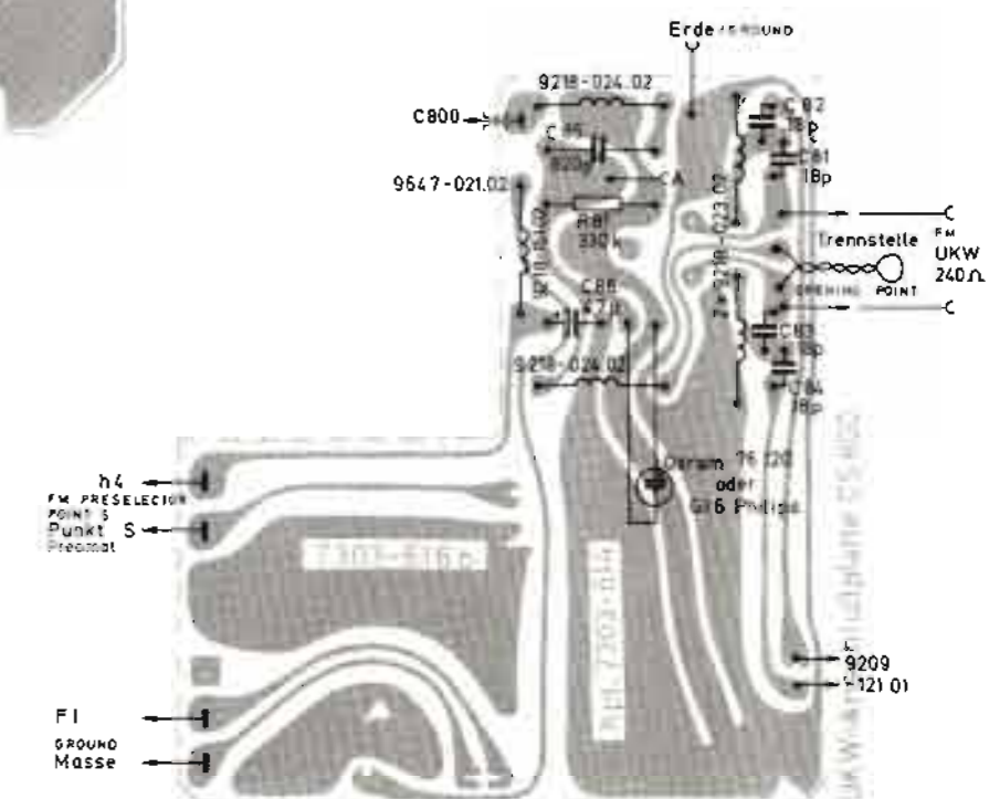
UKW-Anschlußplatte, Lötseite FM CONNECTION BOARD, SOLDER SIDE PLAQUE DE CONNEXION FM, COTE SOUDURES PIASTRA DI COLLEGAMENTO FM, LATO SALDATURE
