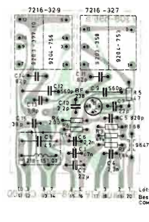
Lötseite / SOLDER SIDE Bestückungsseite COMP. SIDE
