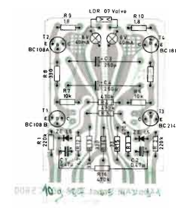
56 V-Platte, Lötseite 56 V PRINTED BOARD, SOLDER SIDE PLAQUETTE 56 V, VUE DU COTE DES SOUDURES PIASTRA 56 V, LATO SALDATURE
